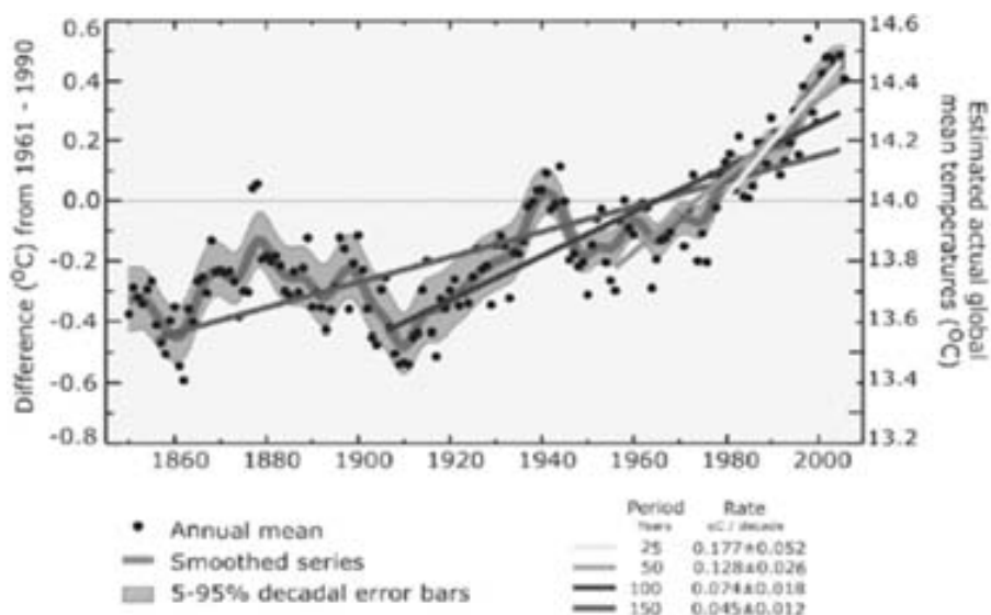
Figura 1 – Evolução da Temperatura Global Média – de 1850 a anos 2000.
