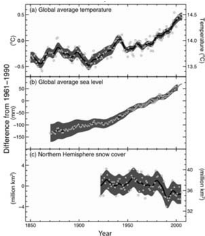
Figura 4 – Evolução Global Média da Temperatura e do Nível do Mar; e da Cobertura de Neve no Hemisfério Norte
