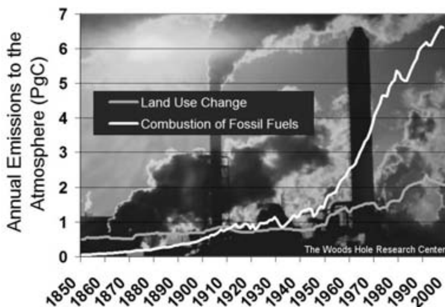
Figura 4 – Emissão de CO 2 de Mudanças de Uso do Solo e Uso de Combustíveis Fósseis – 1850-2000.
