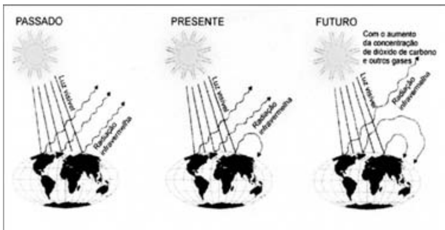
Figura 2 – Como ocorre o Aquecimento Global*
